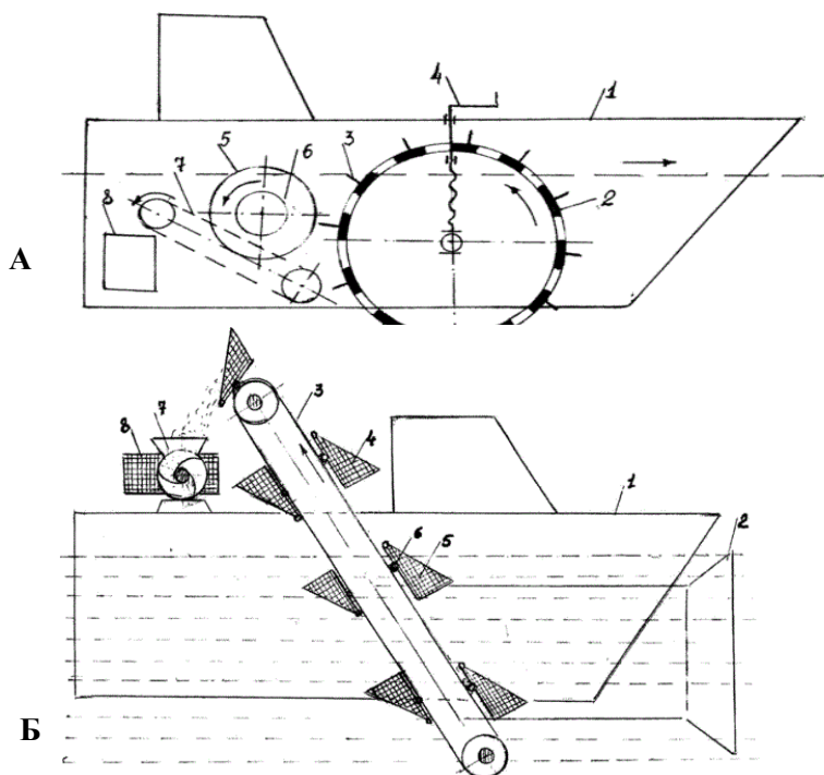
Рис. 2. А Устройства для сбора сине-зеленых водорослей [7]: 1-плавсредство; 2-барабан с зацепами-3; 4-винтовой механизм; 5-барабан-кассета; 6-съемная кассета; 7-транспортёр; 8-контейнер; Б агрегат для очистки водоемов от водорослей [8]: 1-плавсредство; 2-приспособление для водного потока с водорослями; 3-транспортёр; 4-ковши-черпалки; 5-сетка; 6-шарнир; 7-шнек; 8-контейнер.
