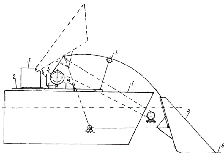
Рис. 1. Устройство для сбора донных отложений [6]: 1-плавсредство; 2-рама; 3-лебедка-; 4-реверс; 5-ковш с зубьями-6; 7-бункер-накопитель; 9-упор.
